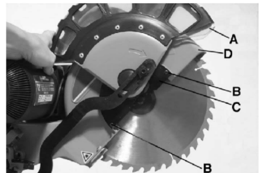
Obr. 13: Demontáž ochranného krytu
