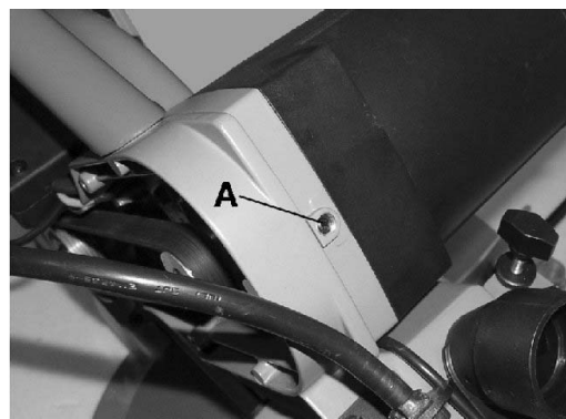
Obr. 18: Napínací šroub klínového řemene
