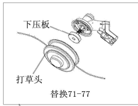
打草头安装图
